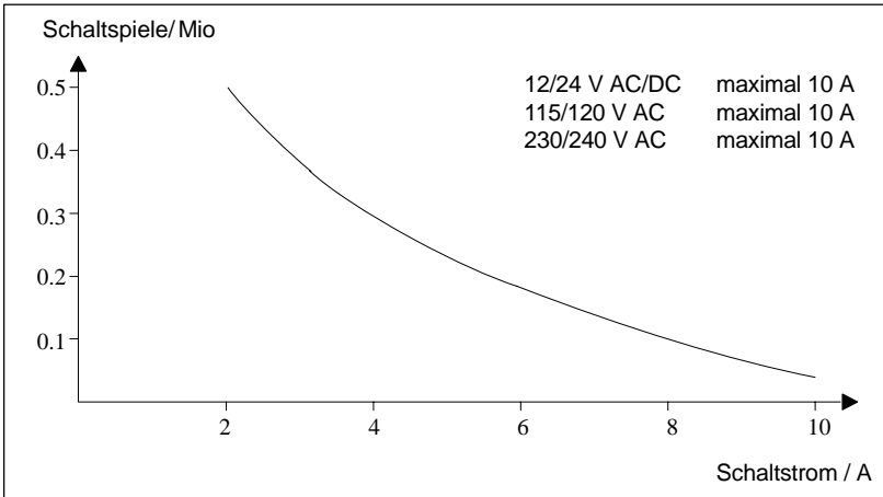
Bild A Schaltvermögen und Lebensdauer der Kontakte bei ohmscher Last (Heizung)
