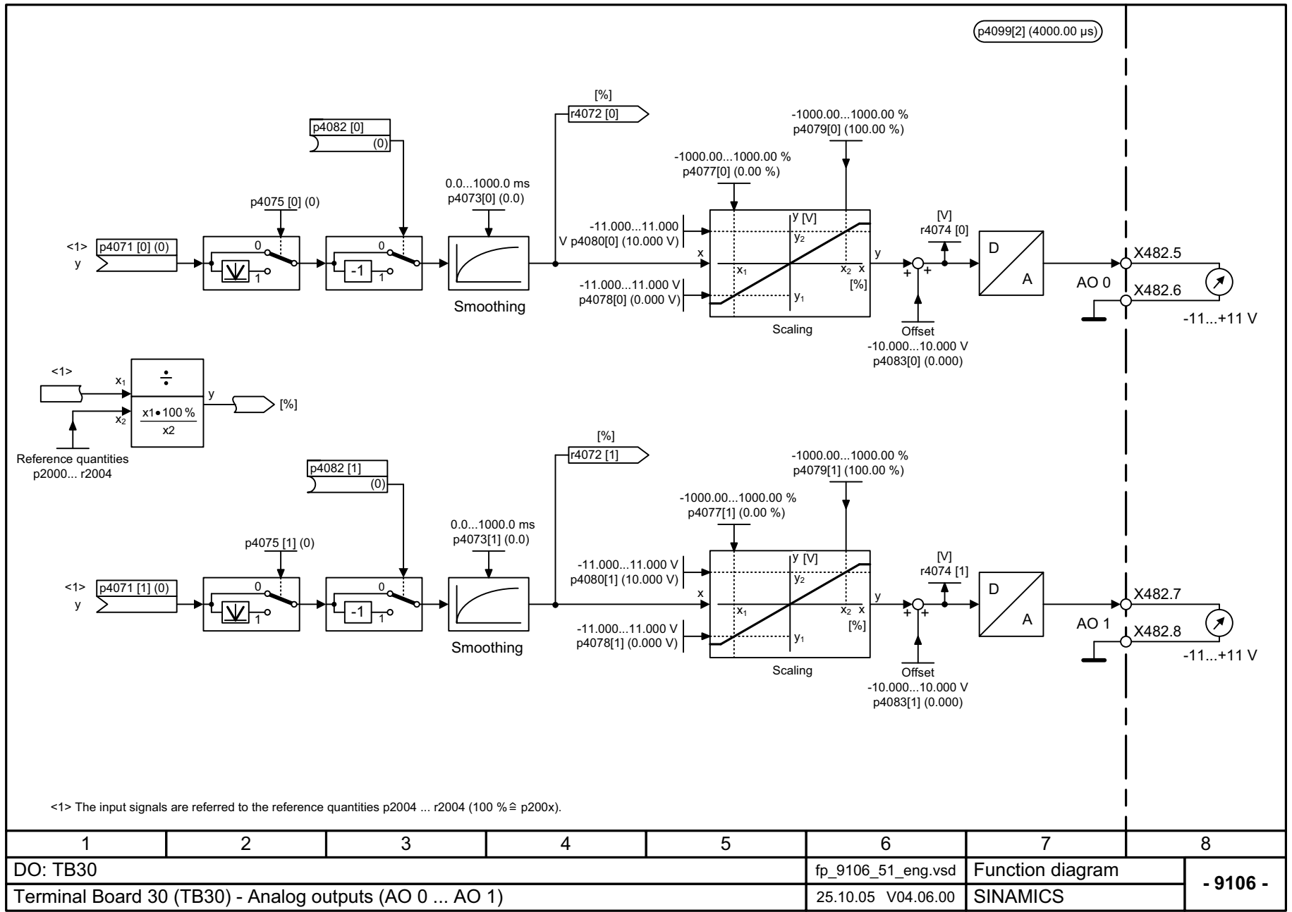
Fig. 2-183 9106 – Analog outputs (AO 0 ... AO 1)
