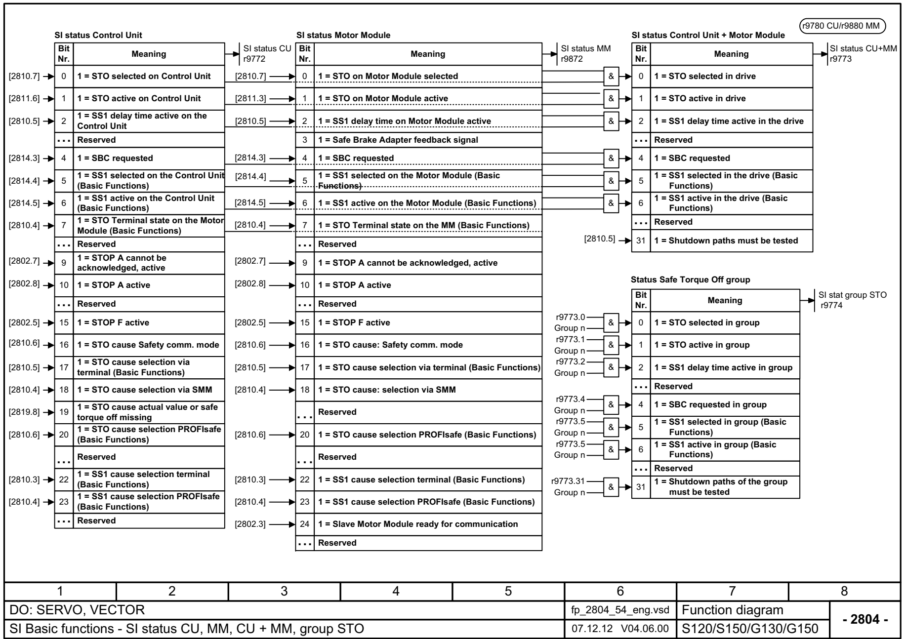
Fig. 2-88 2804 – SI status CU, MM, CU + MM, group STO
