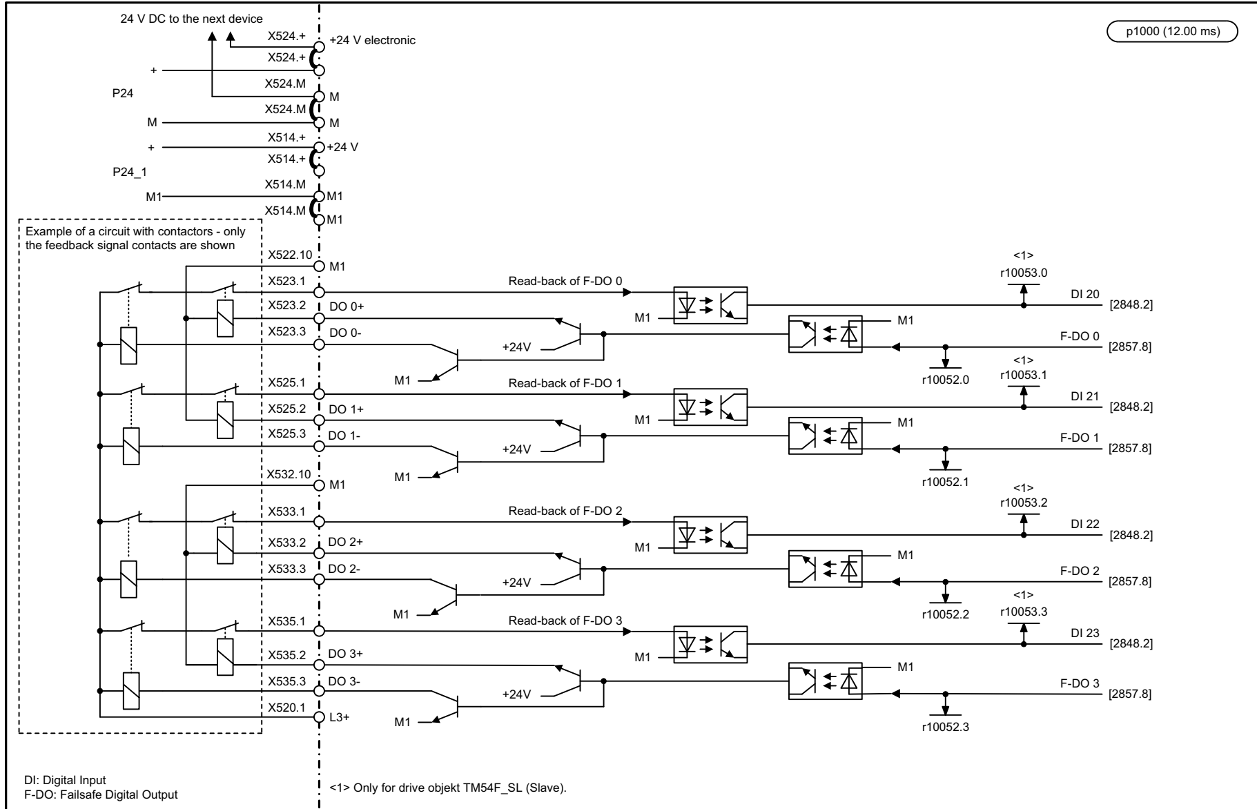
Fig. 2-108 2853 - TM54F (F-DO 0 ... F-DO 3, DI 20 ... DI 23)
