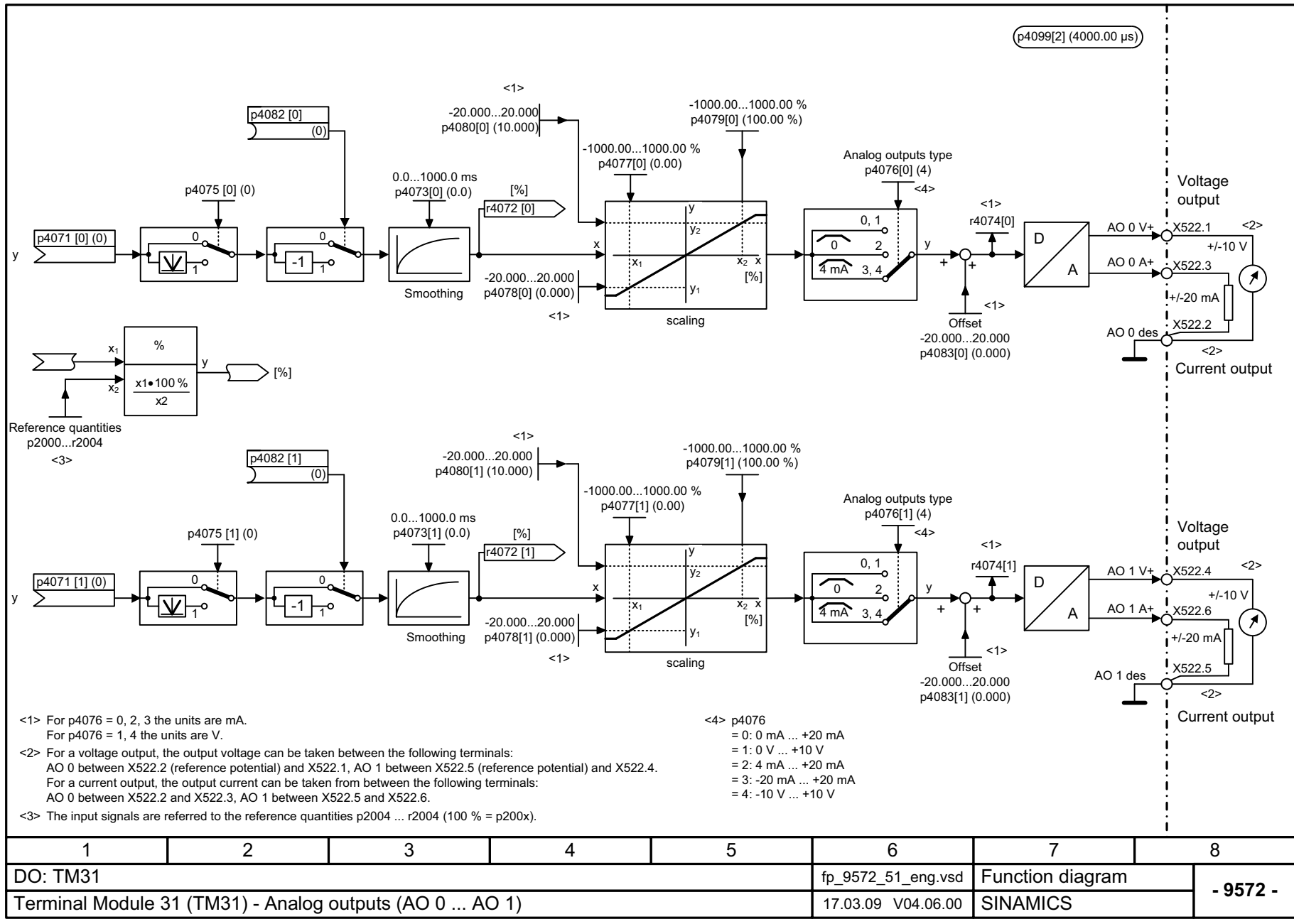
Fig. 2-197 9572 – Analog outputs (AO 0 ... AO 1)
