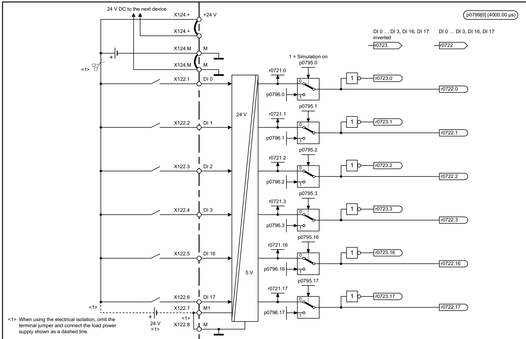
Fig. 2-18 2120 – Digital inputs, electrically isolated (DI 0 ... DI 3, DI 16, DI 17)
