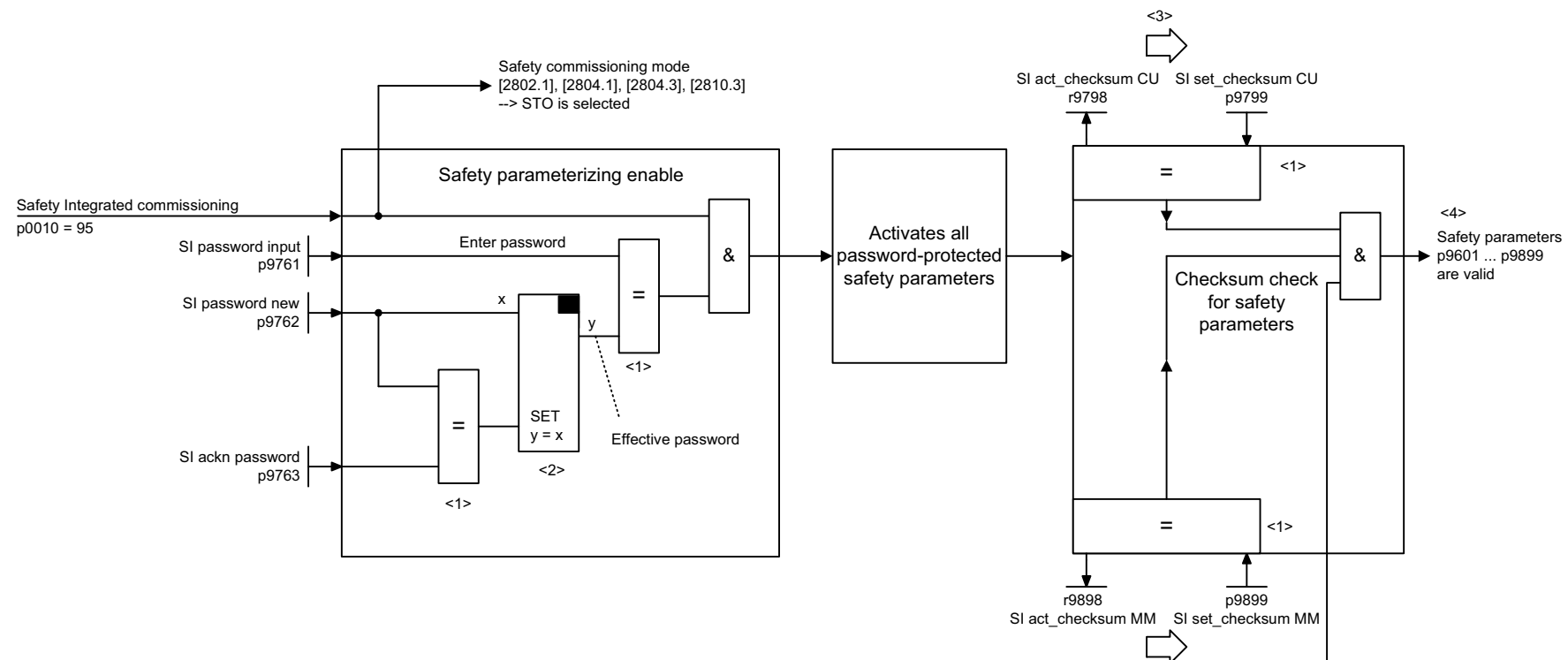
Fig. 2-86 2800 – Parameter manager
