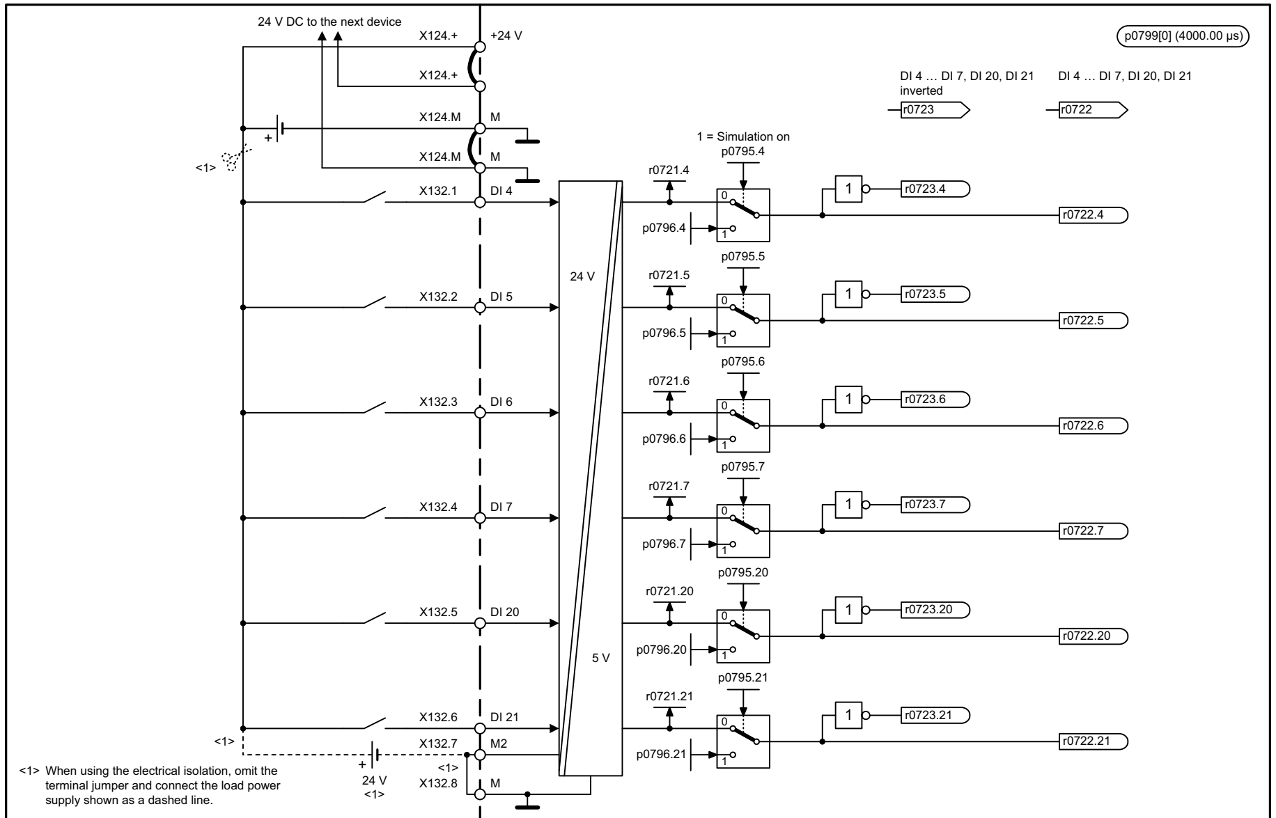
Fig. 2-19 2121 – Digital inputs, electrically isolated (DI 4 ... DI 7, DI 20, DI 21)
