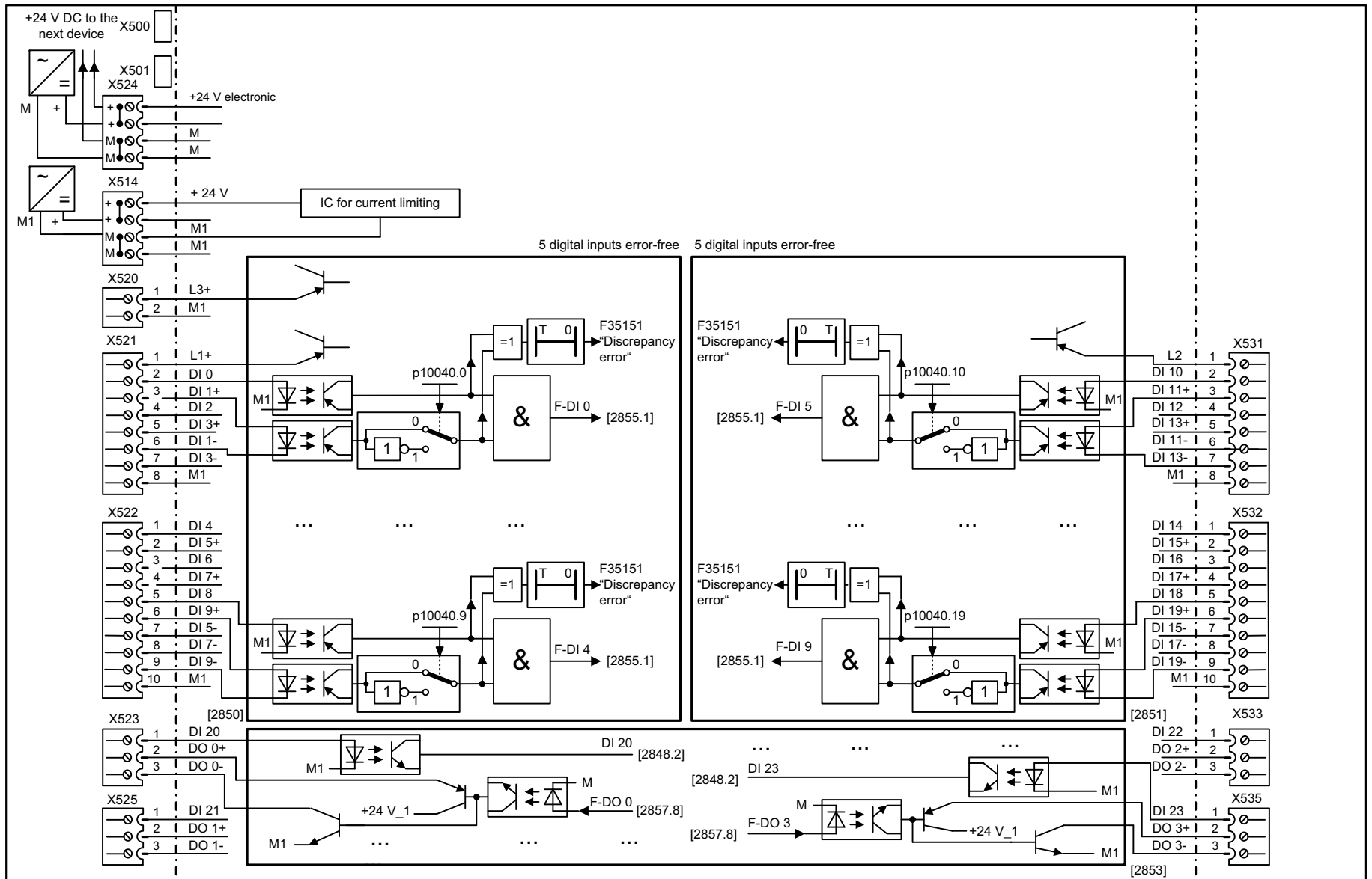
Fig. 2-17 1850 – Terminal Module 54F (TM54F)
