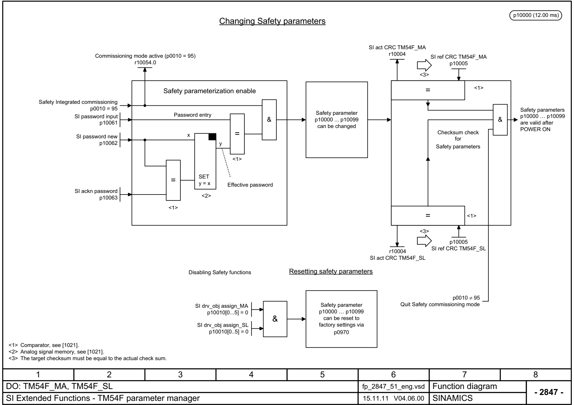
Fig. 2-104 2847 – TM54F parameter manager
