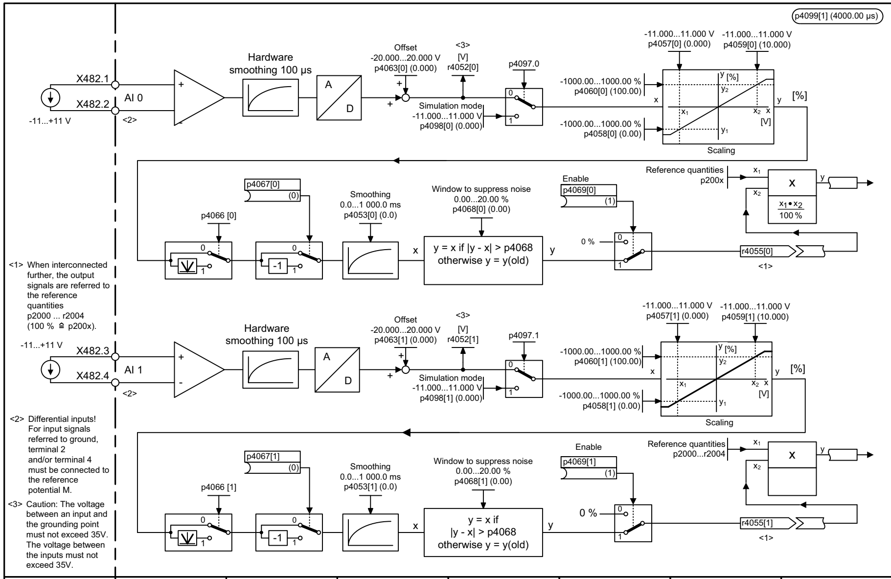
Fig. 2-182 9104 – Analog inputs (AI 0 ... AI 1)
