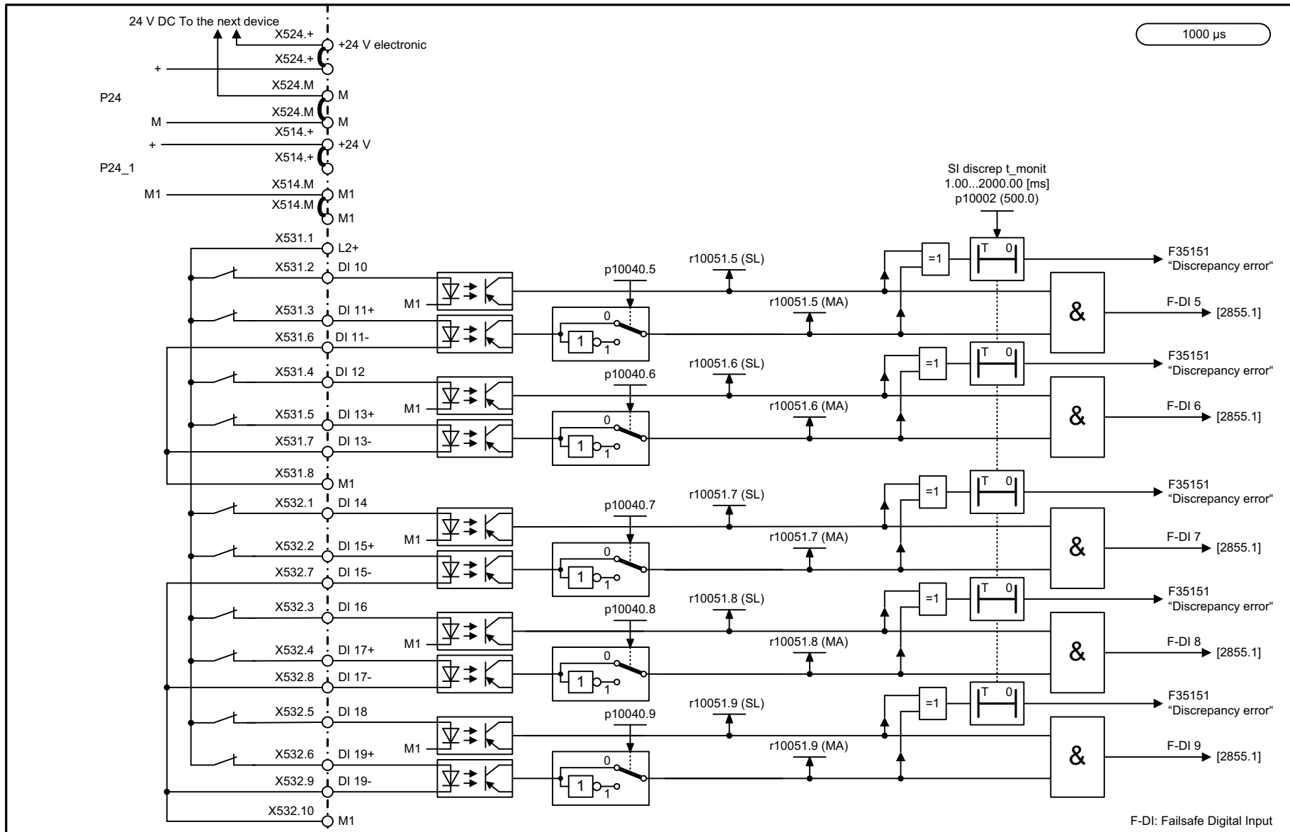
Fig. 2-107 2851 – TM54F (F-DI 5 ... F-DI 9)
