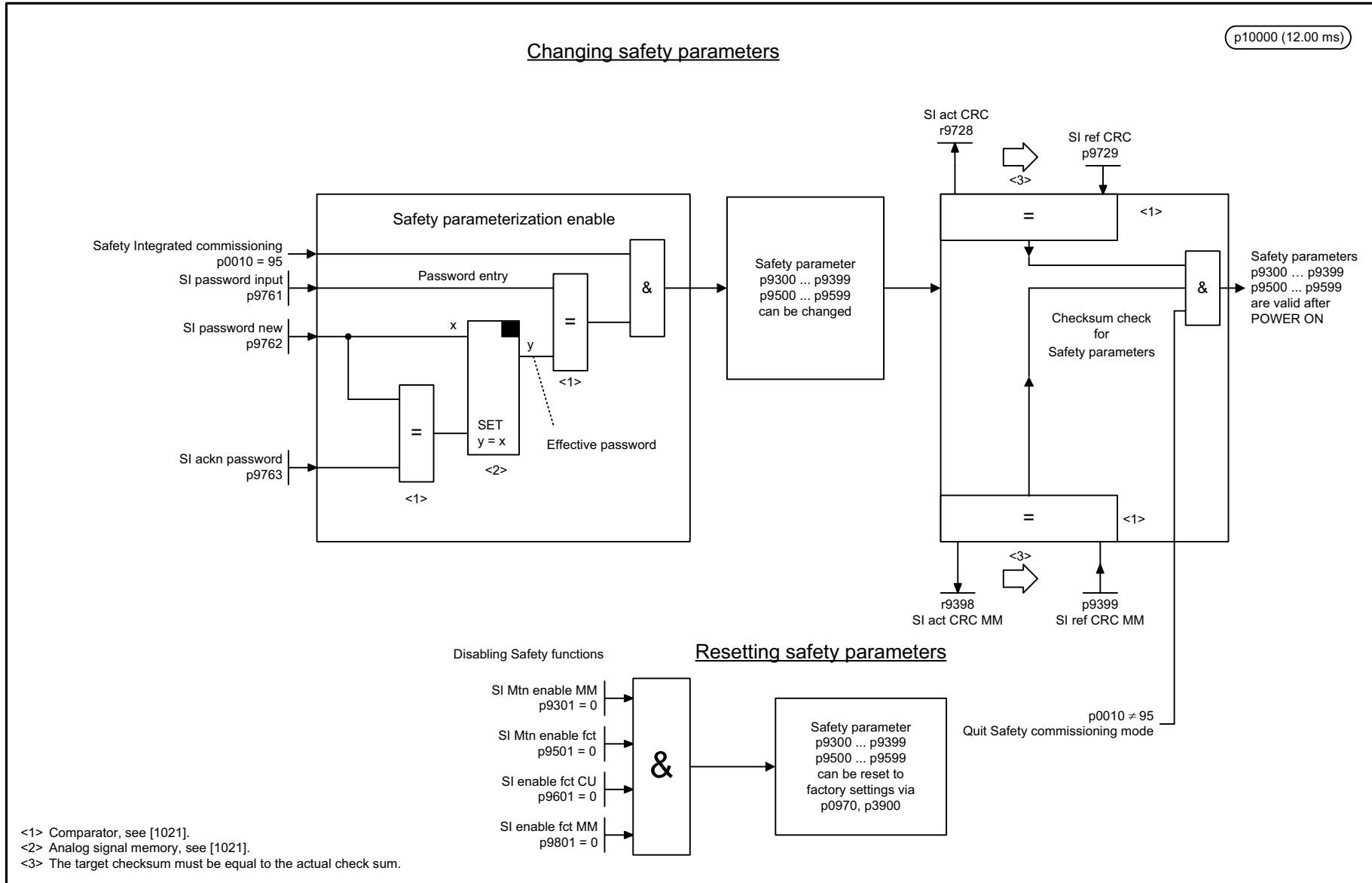
Fig. 2-93 2818 – Parameter manager
