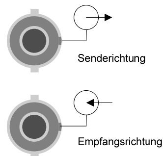
Belegung opt. Port Kanal 2 / Kanal 3
