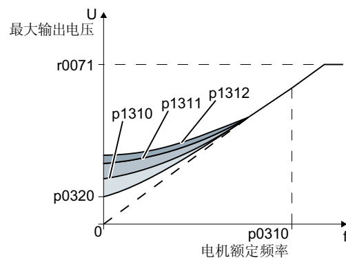
图 8-105 线性特性曲线上的升压降低示例
