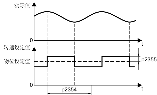
图 8-86 自动优化时的转速设定值和过程实际值示例 变频器根据测得的振动频率计算 PID 控制器的参数。
