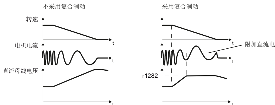
图 8-161 电机制动：无复合制动，有复合制动
