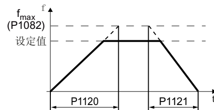
图 5-8 电机的斜坡上升和下降时间
