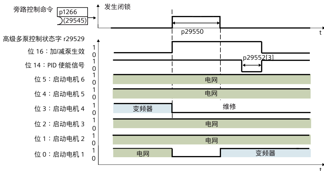
图 8-64 维修模式 - 无闲置电机
