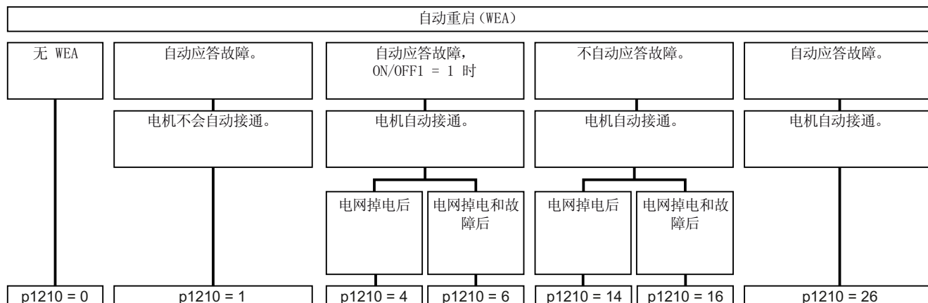
图 8-184 自动重启模式
