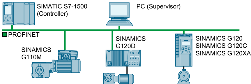
图 4-21 变频器作为 PROFINET IO 设备工作（示例）
