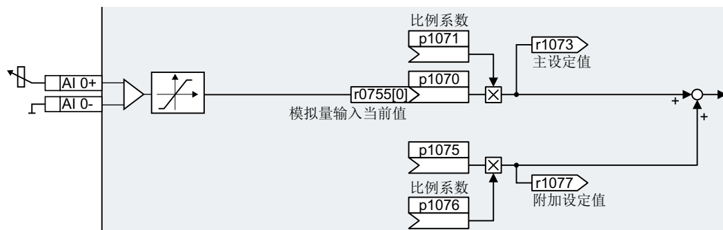
图 8-66 示例：模拟量输入 0 设为设定值源
