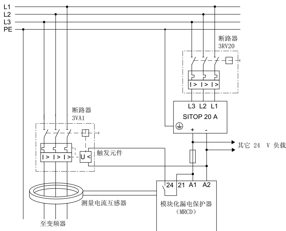
图 4-8 MRCD
