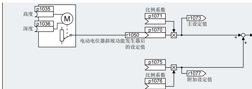
图 8-68 电动电位器设为设定值源
