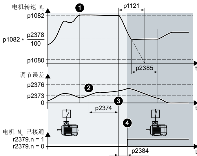
图 8-94 激活非调速电机 M_1 \dots M_2
