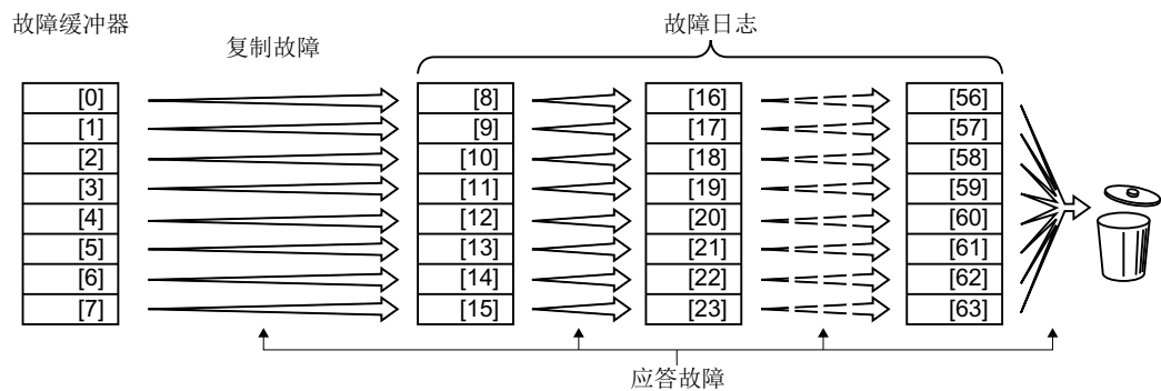
图 10-4 应答故障信息后的故障日志
