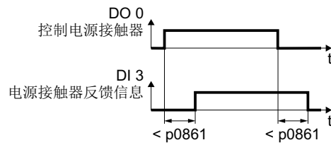
图 8-197 通过 DO 2 的电源接触器控制，带通过 DI 3 的反馈信息
