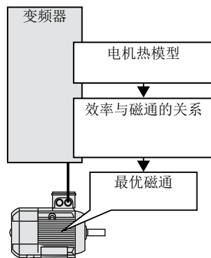
图 8-189 根据电机热模型计算最佳磁通
