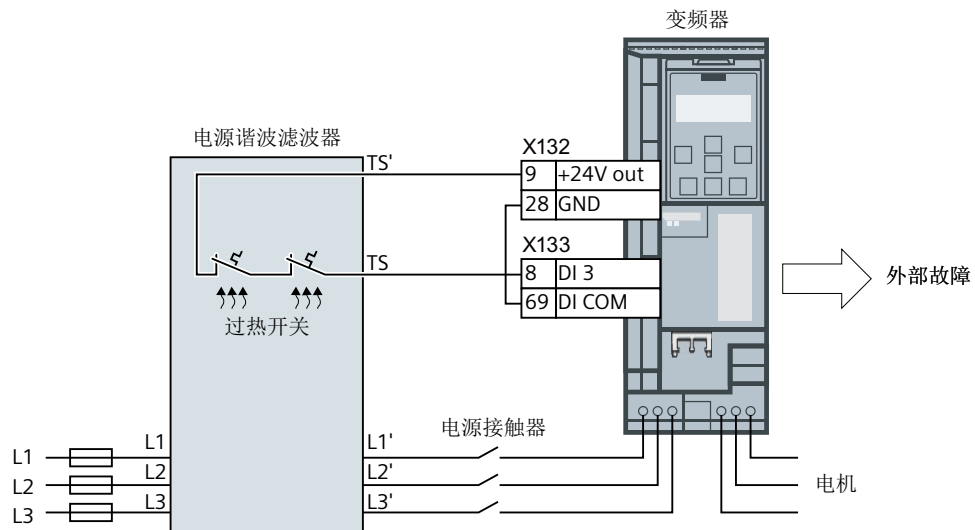
图 2-1 输入谐波滤波器的保护
