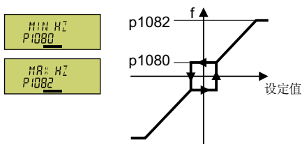
图 5-11 最小和最大电机频率
