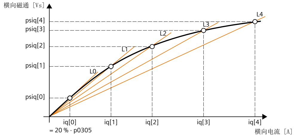
图 8-99 永磁同步电机的饱和特性曲线
