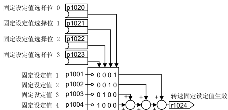
图 8-71 转速固定设定值的直接选择
