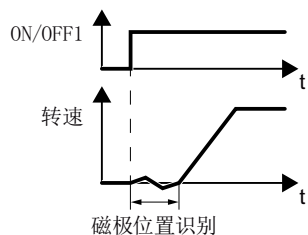
图 8-163 接通电机后检测磁极位置
