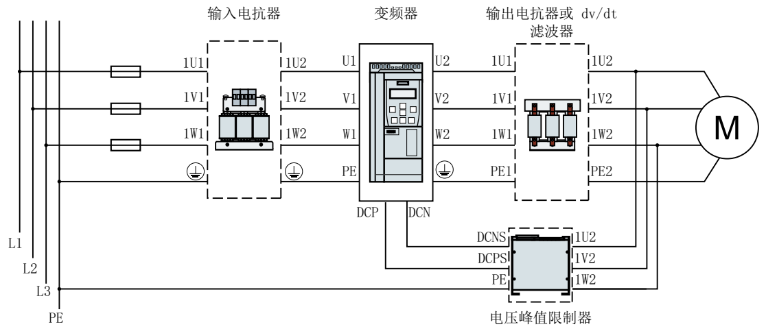
图 4-10 连接变频器 FSH/FSJ 及其选件
