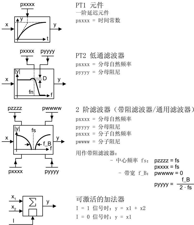
图 8-205 模拟量模块
