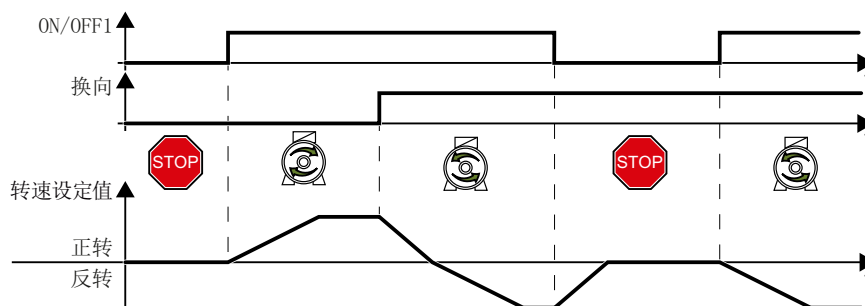
图 8-50 双线制控制，ON/换向
