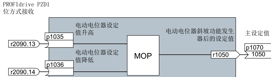
图 8-207 示例：数字量输入 0 上两个功能块的信号互联
