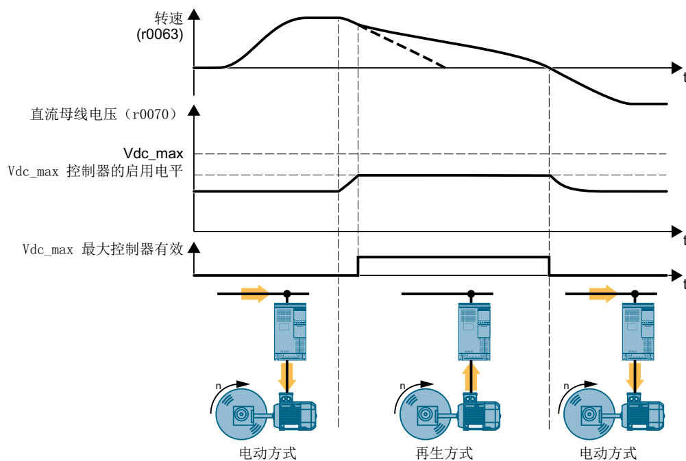
图 8-168 最大 V_{dc} 控制器的简化图
