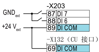
图 2-3 连接漏型触点
