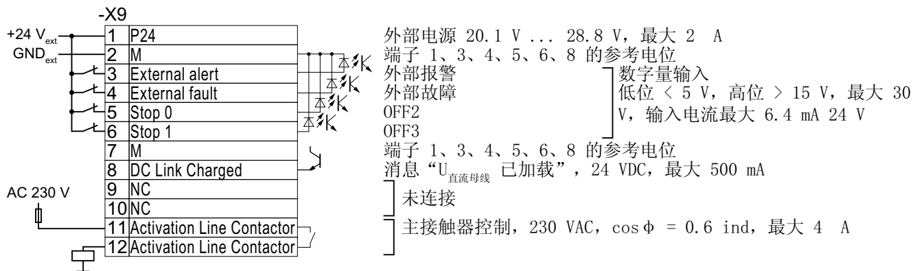
图 4-19 连接外部 24 V 电源
