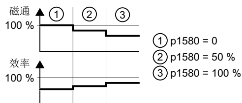
图 8-192 效率优化，方法 1 的结果
