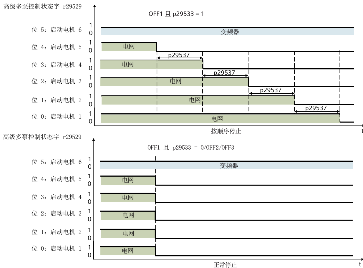
图 8-61 停机模式
