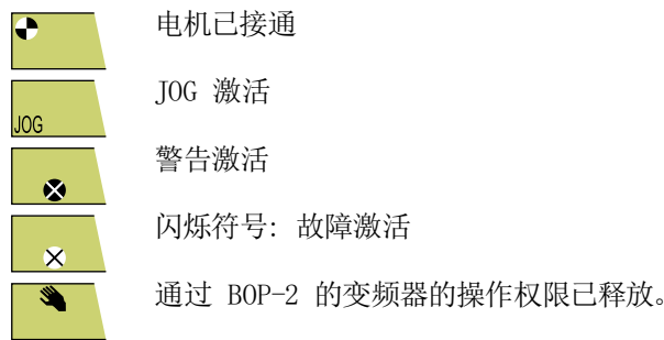
图 5-14 BOP-2 的其他符号
