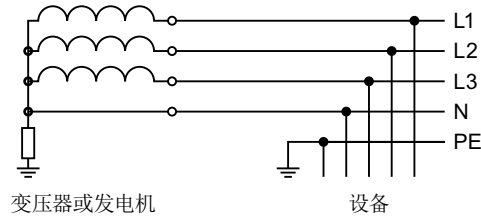
图 4-7 IT 系统
