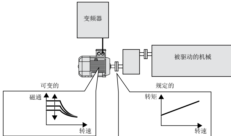
图 8-188 通过改变电机磁通实现效率优化
