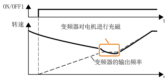
图 8-183 “捕捉重启”功能的工作原理
