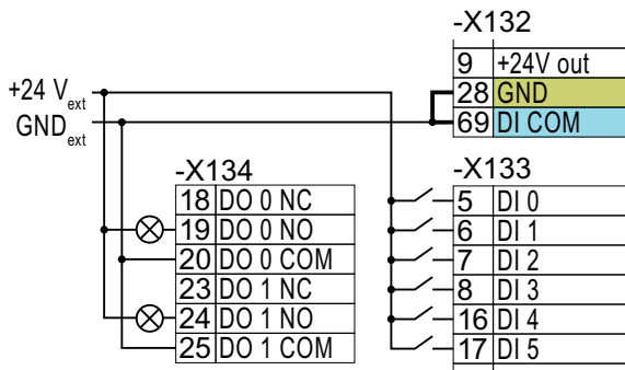
图 4-16 将源型触点连接到外部电源
