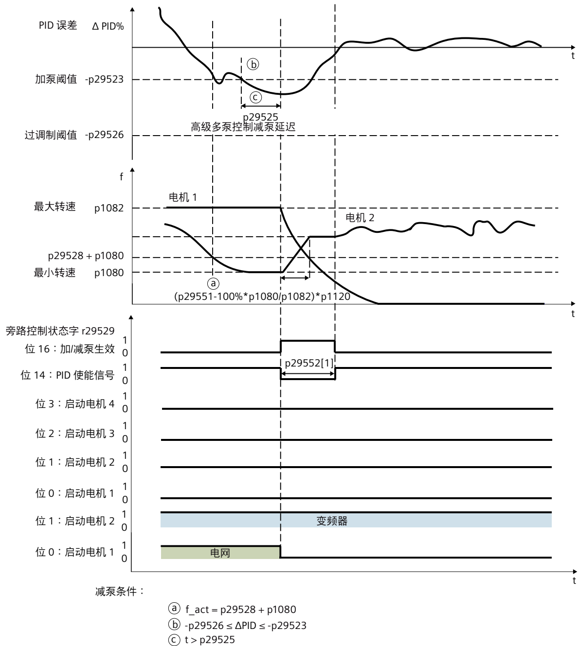
图 8-60 减泵
