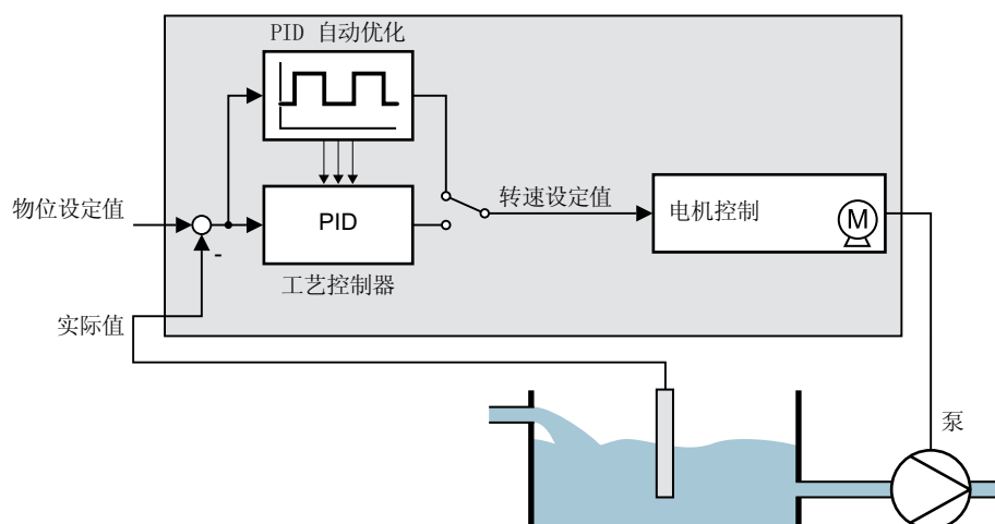
图 8-85 自动优化示例（物位调节）
