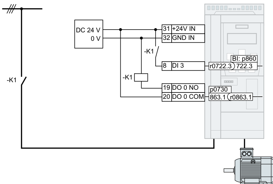
图 8-196 通过 DO 0 的电源接触器控制，带通过 DI 3 的反馈信息
