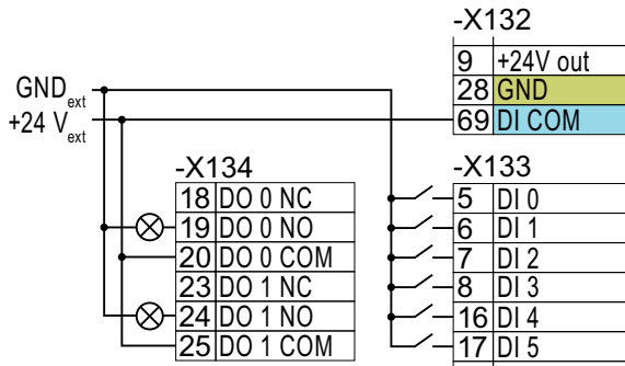
图 4-17 将漏型触点连接到外部电源
