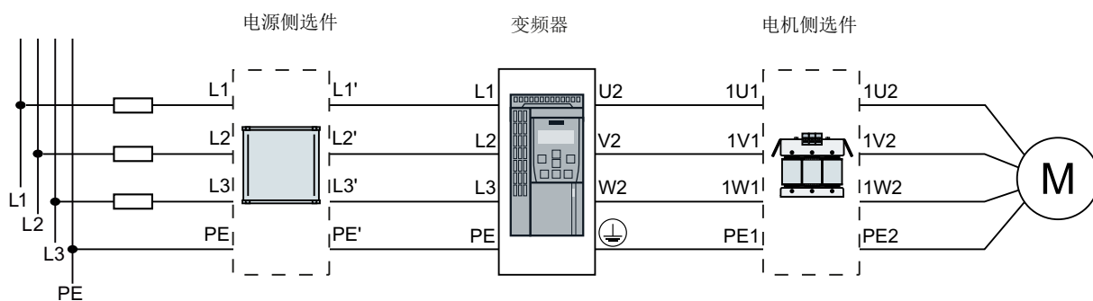
图 4-9 连接变频器 FSA ... FSG 及其选件
