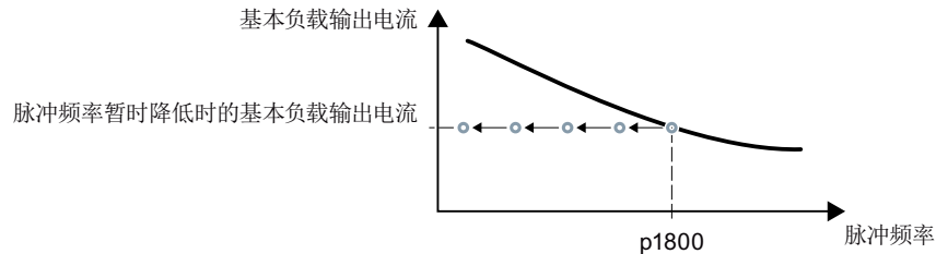
图 8-164 过载时的降容特性曲线和基本负载输出电流
