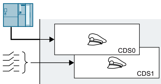
图 8-34 通过现场总线或端子排控制变频器
