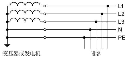
图 4-5 TN 系统
