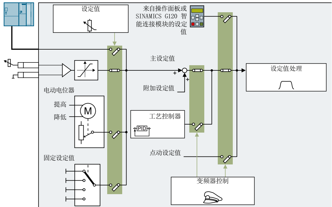
图 8-65 变频器的设定值源
