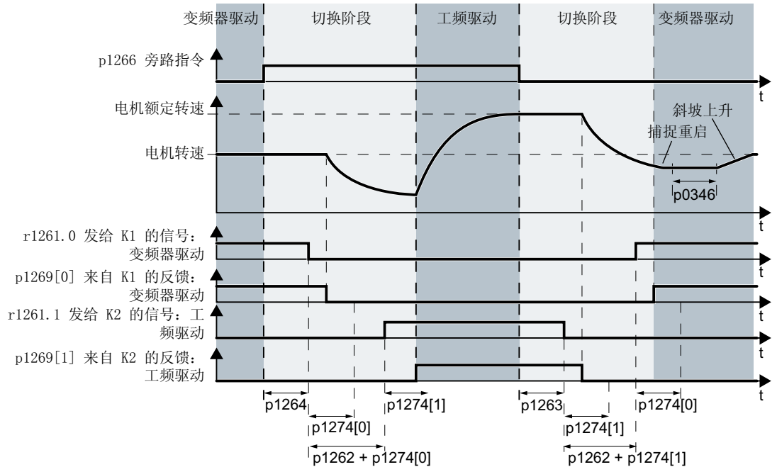
图 8-194 通过控制信号激活时切换 (p1267.0 = 1)
