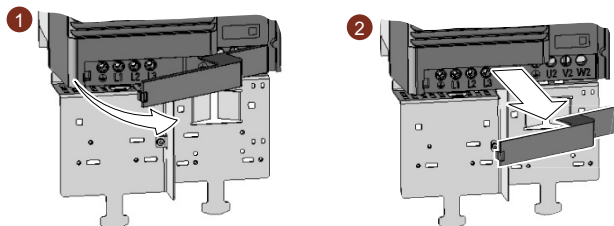
图 4-11 拆除接口盖板，FSD/FSE
