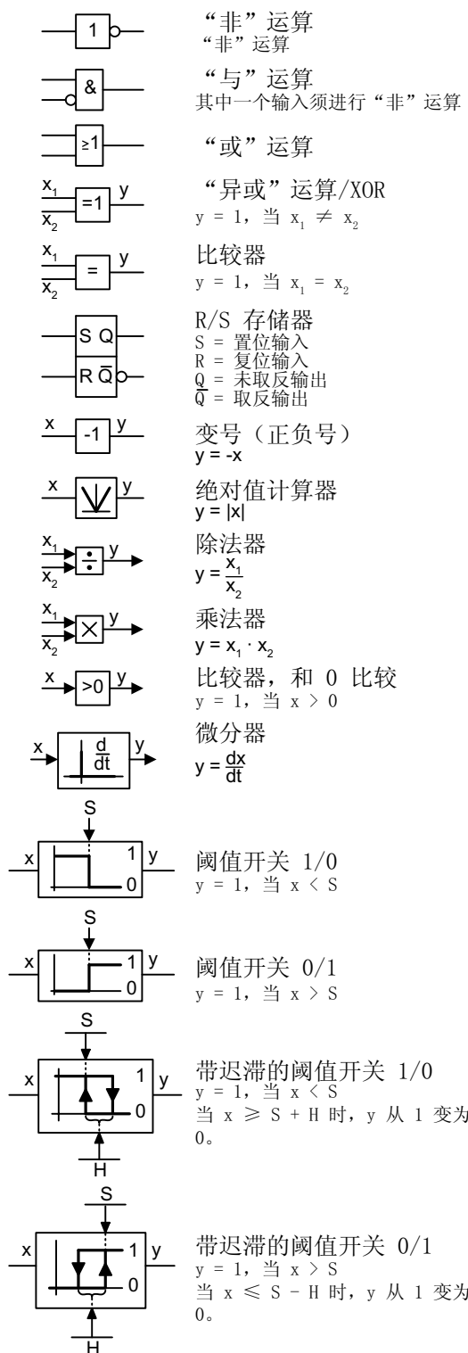
图 8-204 二进制和模拟量模块
