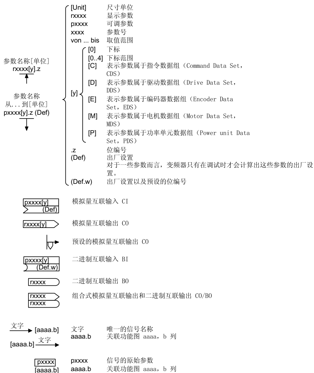
图 8-203 参数
