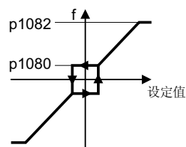
图 5-9 电机的最小频率和最大频率
