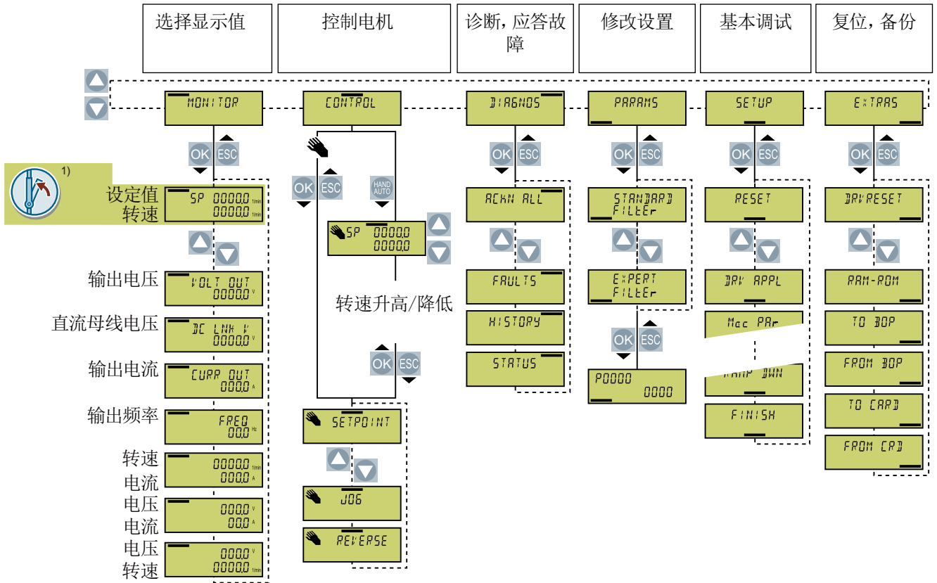
图 5-13 BOP-2 的菜单
