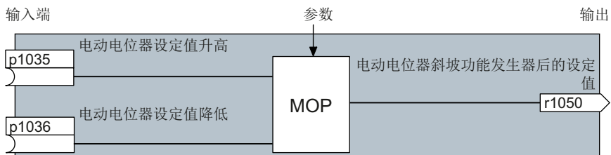
图 8-206 功能块的示例: 电动电位器 (MOP)
