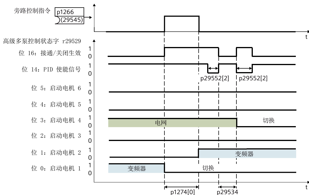
图 8-62 多泵轮换
