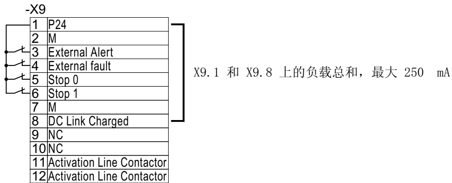
图 4-20 连接内部 24 V 电源
