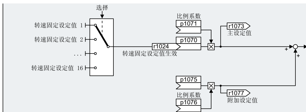
图 8-70 转速固定设定值设为设定值源
