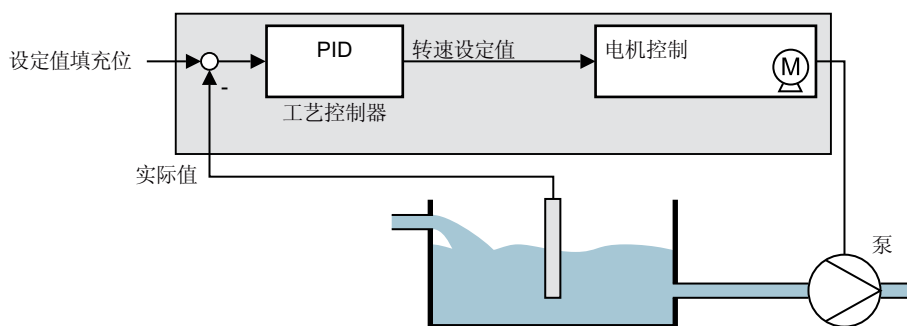
图 8-83 示例：工艺控制器用作流量控制器
