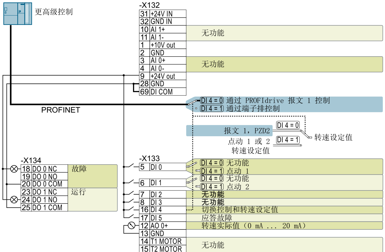
图 4-18 带 PROFINET 接口的变频器的出厂设置
