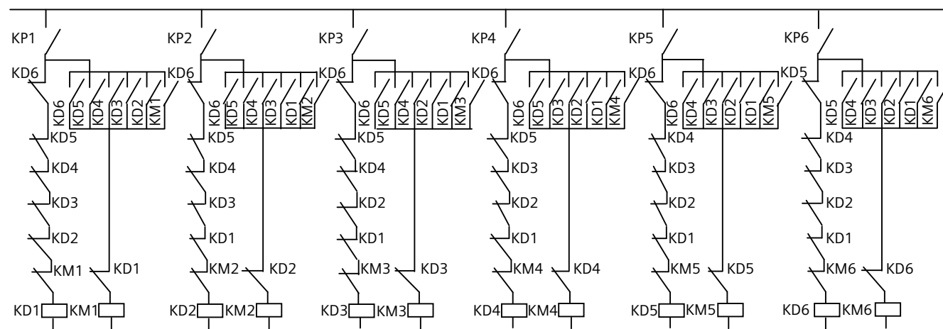
图 8-58 外部继电器控制电路
