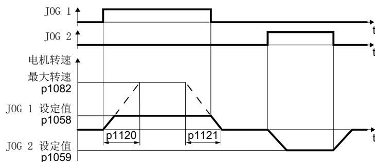
图 8-33 JOG 时电机的工作时序
