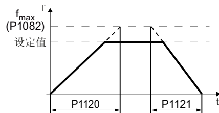
图 5-12 电机的斜坡上升和斜坡下降时间
