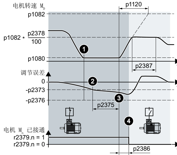
图 8-95 关闭非调速电机 M_1 \dots M_2
