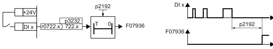
图 8-176 旋转监控的功能图和时序图
