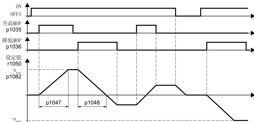
图 8-69 电动电位器的功能图
