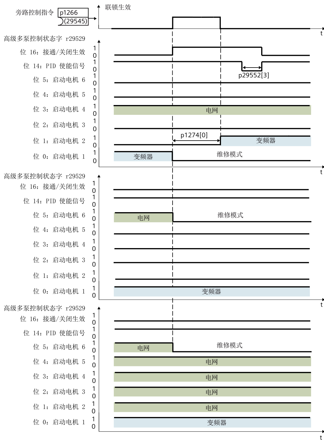
图 8-63 维修模式
