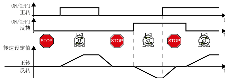
图 8-52 双线制控制, 正转/反转
