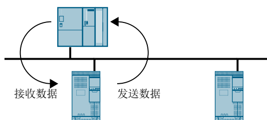
图 8-11 循环数据交换
