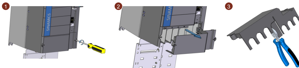
图 4-12 拆除连接盖板并开口，FSF/FSG
