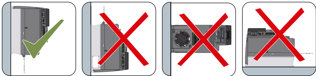
图 3-1 只有在垂直安装时才可使用下方的电源端子
