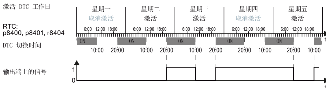
图 8-96 数字时钟的特性示例
