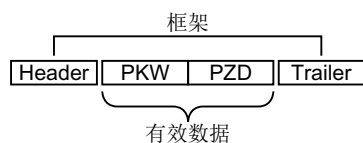
图 8-12 报文结构
