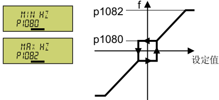
图 5-7 电机的最小频率和最大频率
