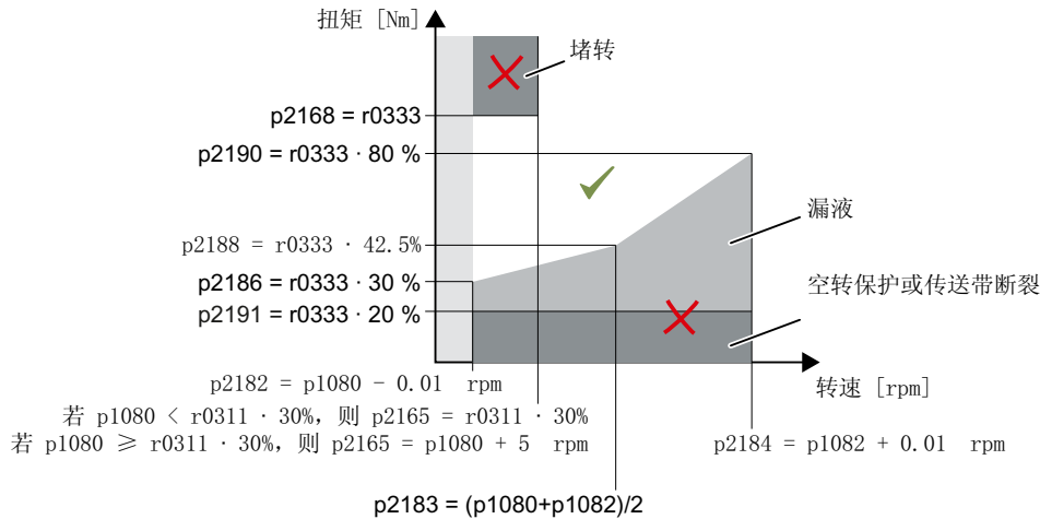
图 8-174 泵应用的预设置
