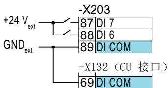
图 2-2 连接源型触点
