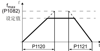
图 5-10 电机的斜坡上升和下降时间
