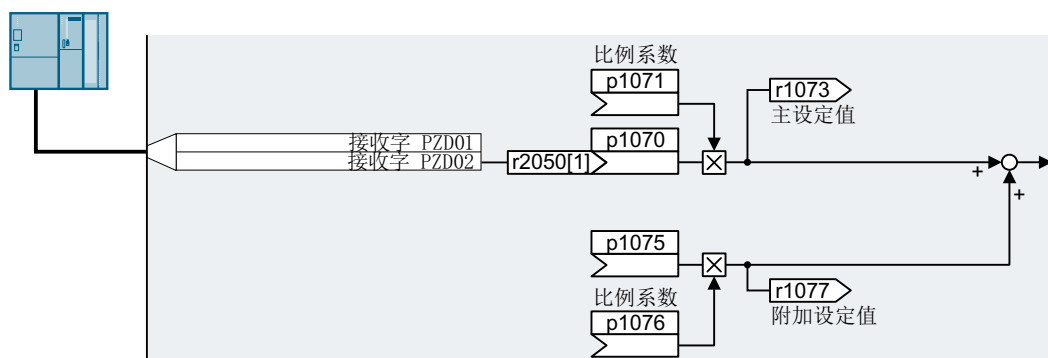
图 8-67 现场总线设为设定值源
