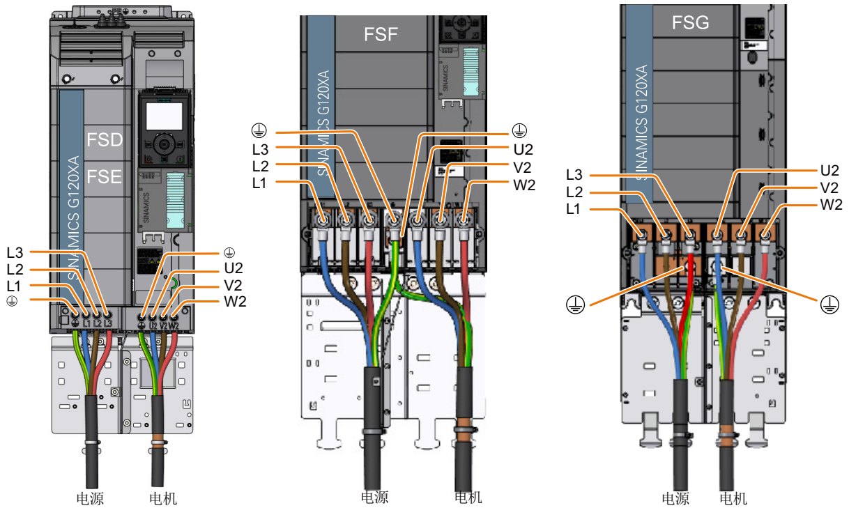
图 4-13 连接电源和电机
