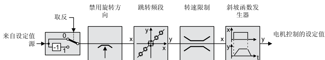
图 8-78 变频器内的设定值处理
