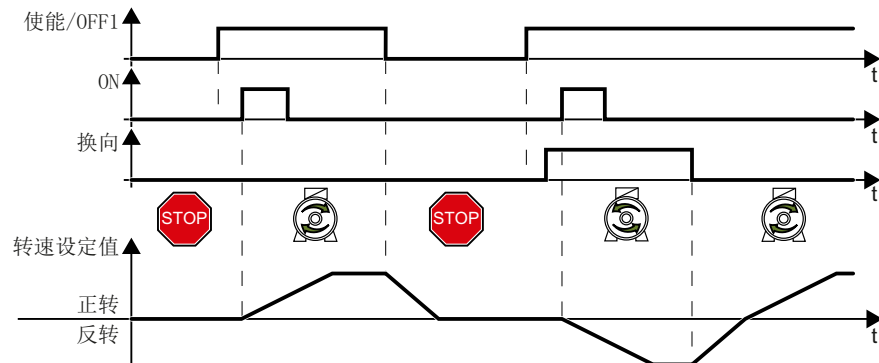
图 8-54 三线制控制，使能/ON/换向
