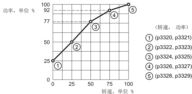
图 8-200 流体特性曲线的出厂设置
