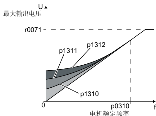
图 8-102 线性特性曲线上电压提升的示例
