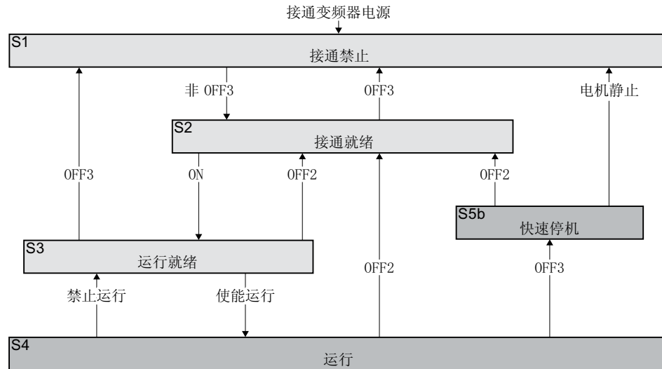
图 8-3 电机接通和关闭时变频器的顺序控制
