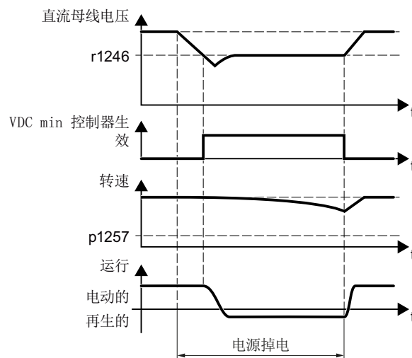
图 8-186 动能缓冲的工作原理
