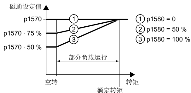
图 8-191 在额定负载以下运行时磁通设定值降低
