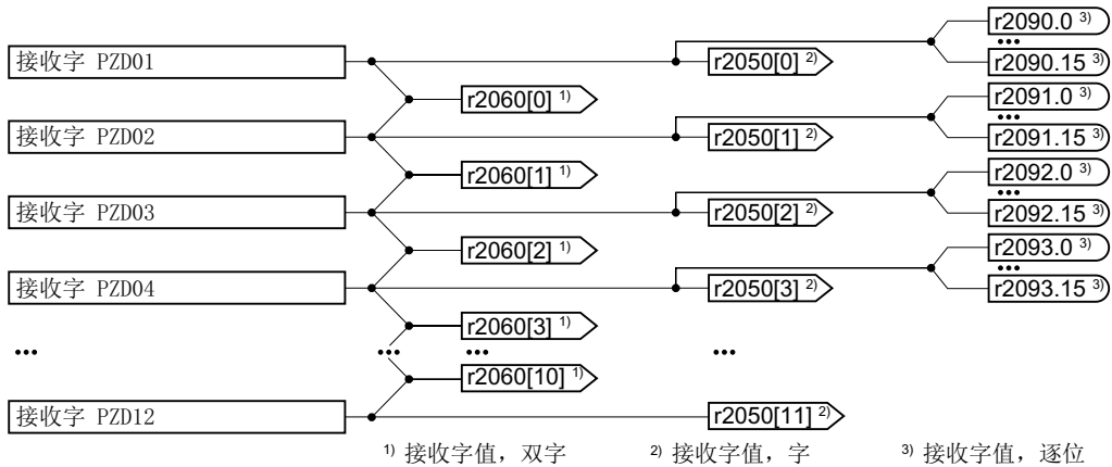
图 8-17 接收数据的互联
