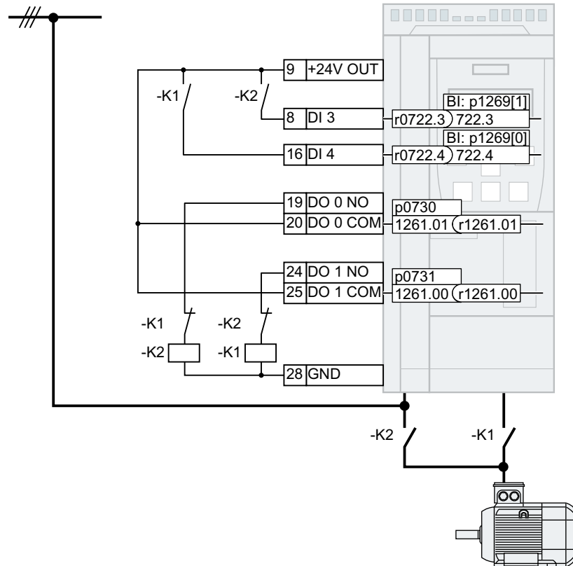
图 8-193 由变频器进行的旁路控制
