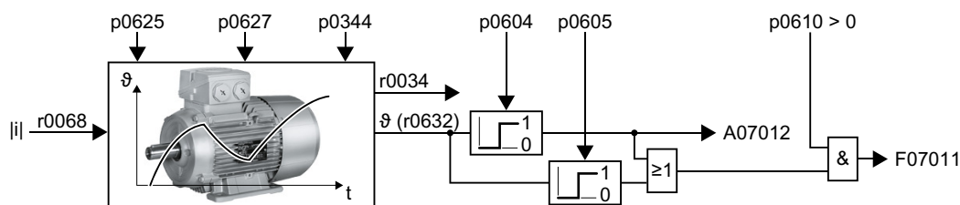
图 8-166 感应电机的热模型 2
