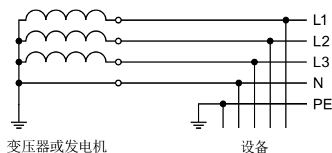
图 4-6 TT 系统
