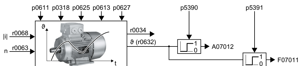
图 8-167 用于磁阻电机的电机热模型 1
