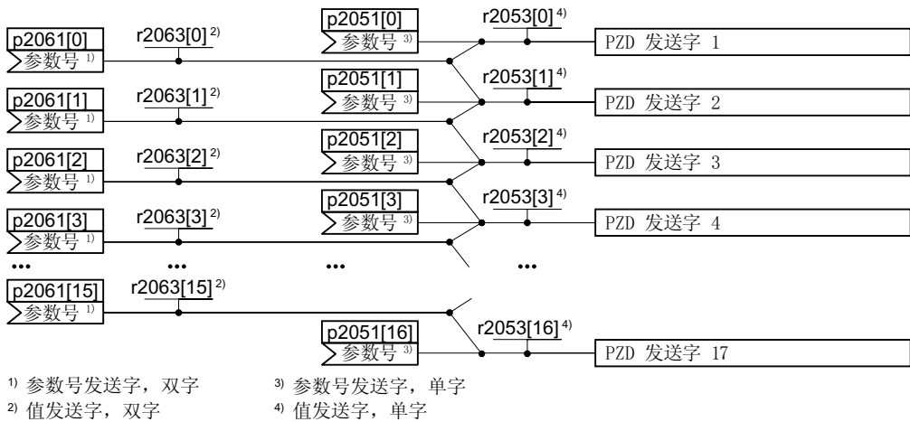
图 8-16 发送数据的互联
