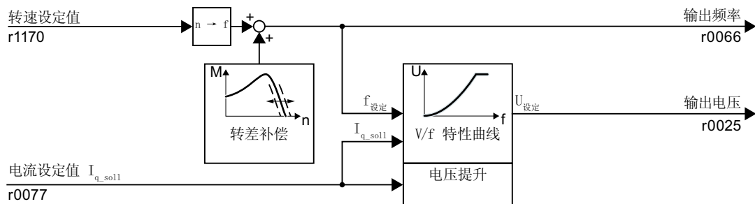
图 8-103 选择 Standard Drive Control 后的 V/f 控制默认设置
