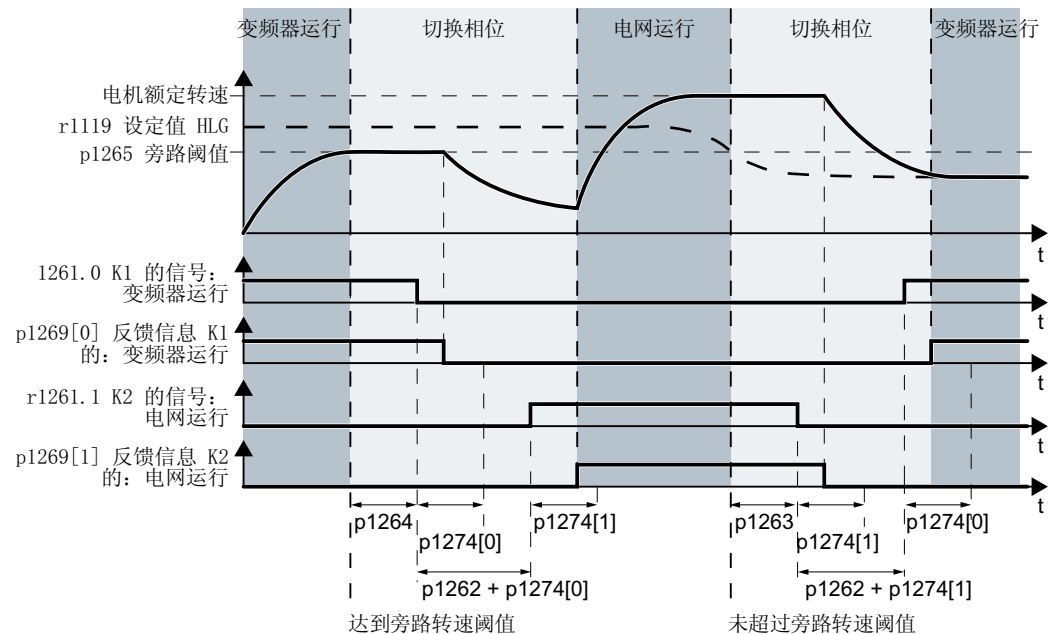
图 8-195 根据转速切换 (p1267.1 = 1)
