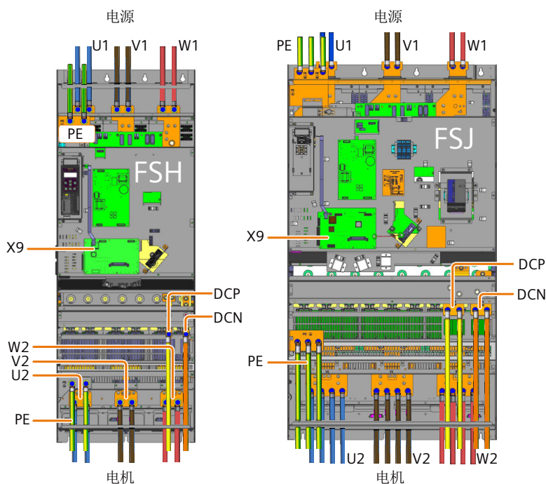
图 4-14 连接电源和电机
