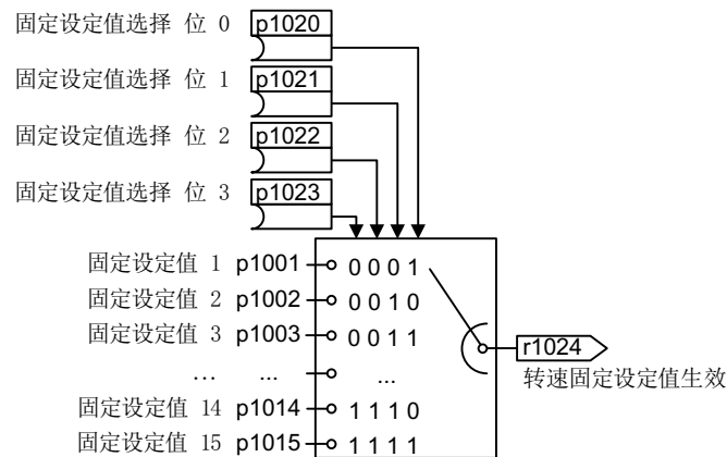
图 8-72 转速固定设定值的二进制选择
