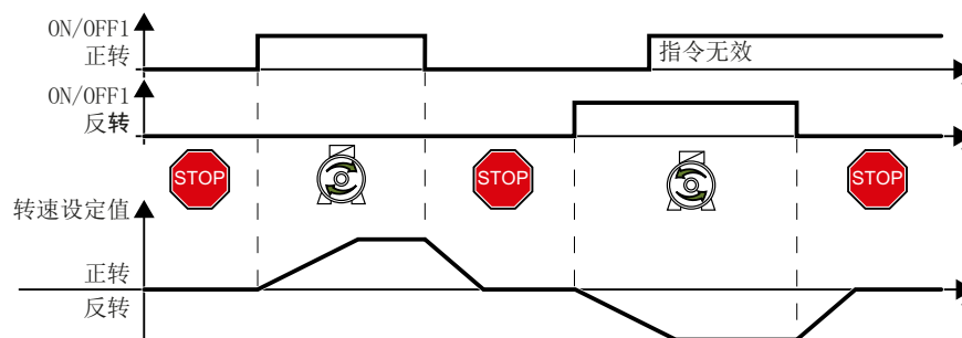
图 8-51 双线制控制，正转/反转 1
