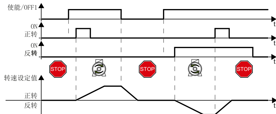
图 8-53 三线制控制，使能/正转/反转
