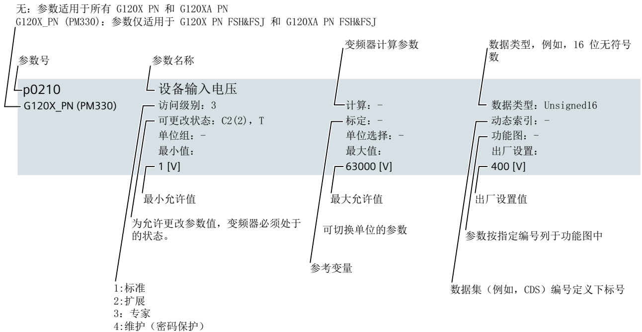
图 9-1 参数说明
