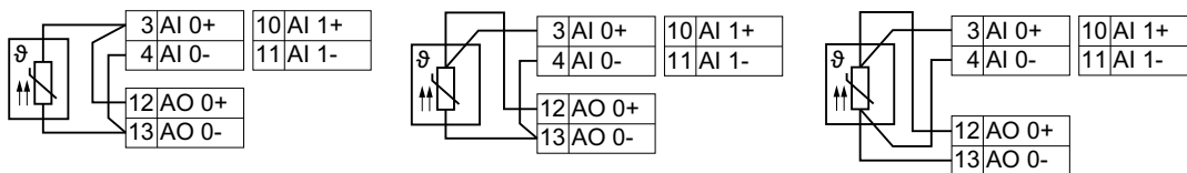
图 8-165 双线制连接、三线制连接和四线制连接
