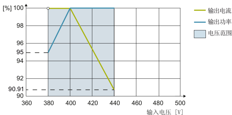
图 12-1 输入电压与电流和电压降容的函数关系
