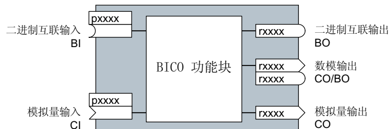
图 8-208 二进制输入/输出和模拟量输入/输出的符号
