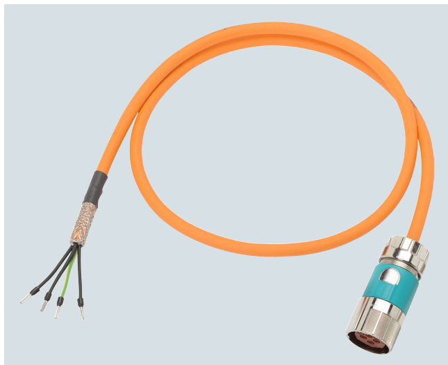
带 SPEED-CONNECT 连接器的 SIMOTICS S-1FK7 电机的动力电缆，连接到 SINAMICS S120 Combi 功率模块上
