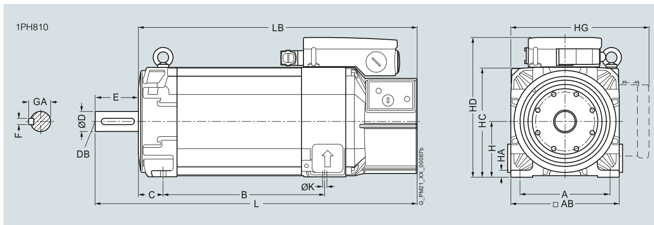
尺寸图
