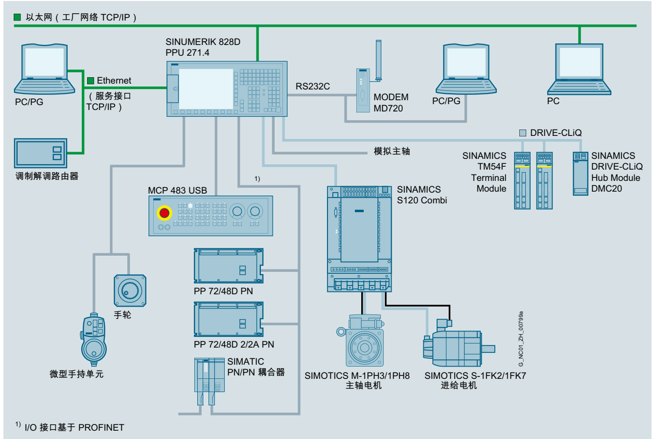
SINUMERIK 828D PPU 271.4 与 SINAMICS S120 Combi 的组态示例
