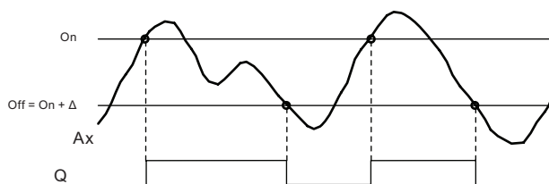
时序图 A: 带有负的差值 \Delta 的功能
