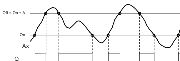
时序图 B: 带有正的差值 \Delta 的功能
