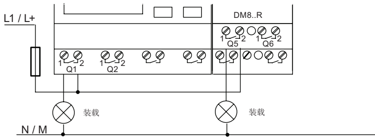
使用自动断路器进行保护，该断路器的最大电流为16 A，特征为B16 例如：电源断路器 5SX2 116-6（如果需要）
